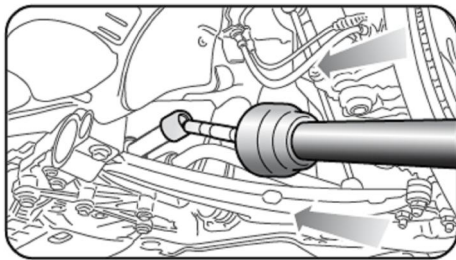
インナー・タイロッド* Assy
